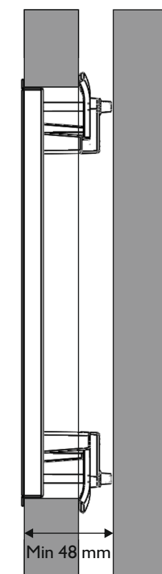
inWall hollow wall
